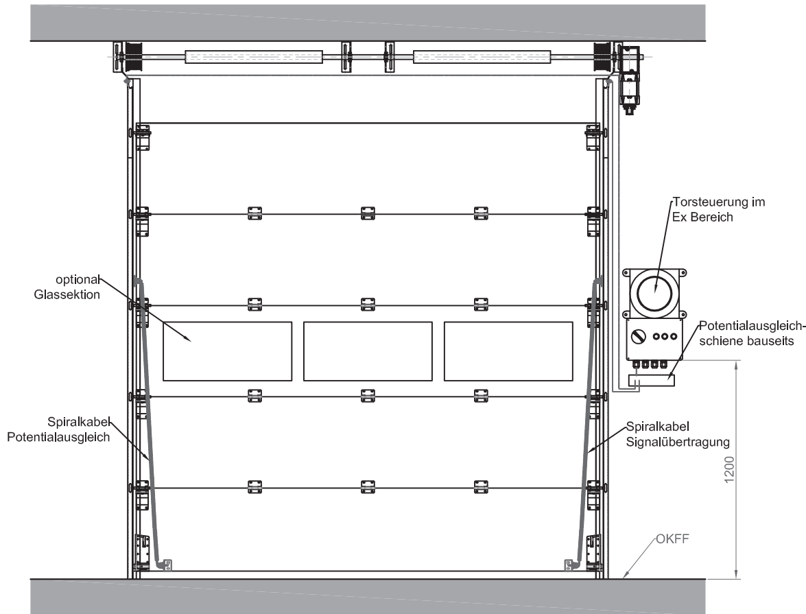
Gesamtansicht Innen
