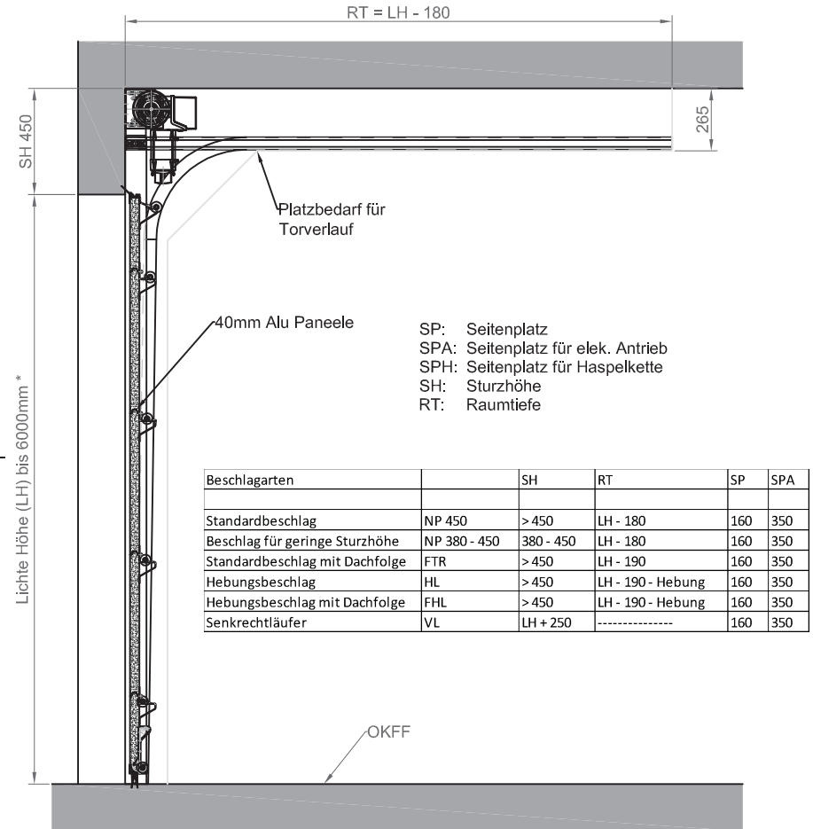
Vertikalschnitt
