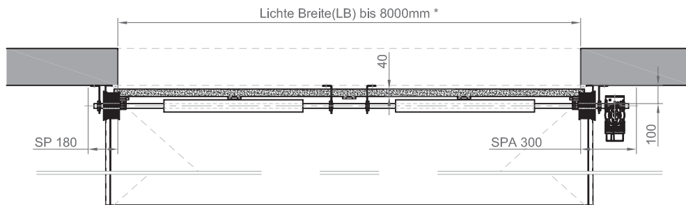
Horizontalschnitt
