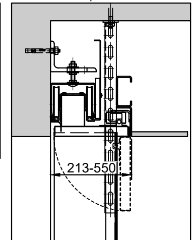
Deckenklappe "optional"
