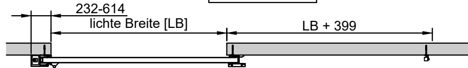
Gegengewicht umgelenkt
