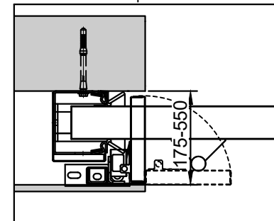
Seitenklappe "optional"
