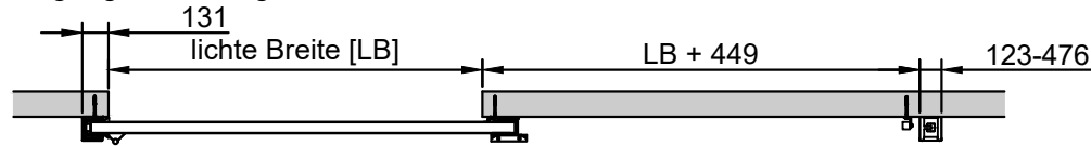
stumpfer Einlauf
