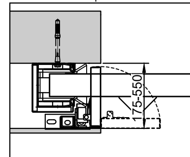
Seitenklappe "optional"
