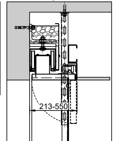
Deckenklappe "optional"
