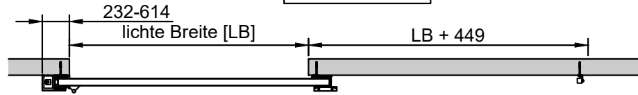
Gegengewicht umgelenkt
