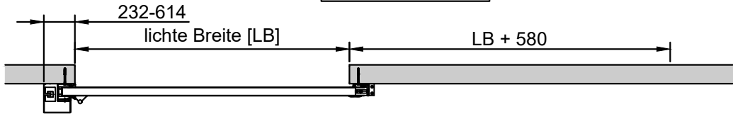
Horizontalschnitt
