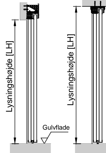
Vertikalt snit
