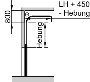
Hebungsbeschlag
