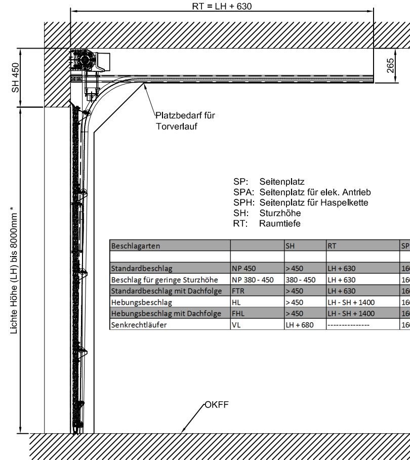
Vertikalschnitt
