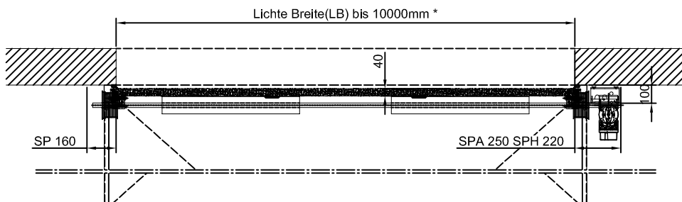
Horizontalschnitt
