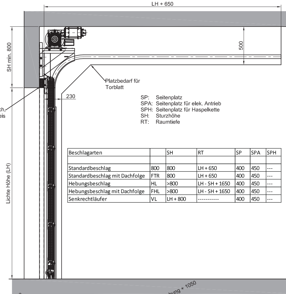
Vertikalschnitt
