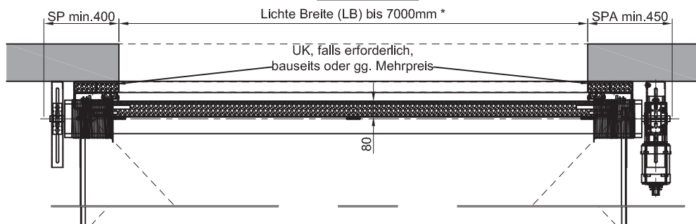
Horizontalschnitt
